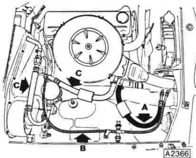
Anordnung Leitungsverlegungen
