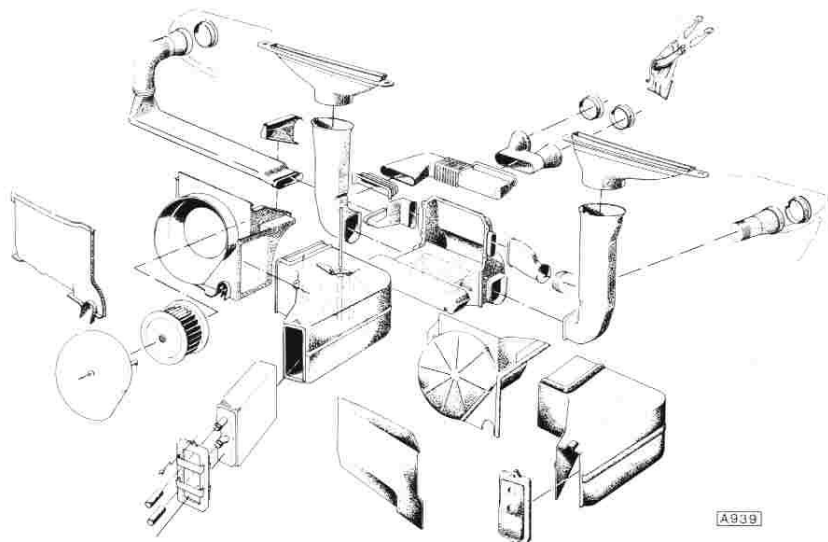
Anordnung der Heizungs- und Lüftungsteile
